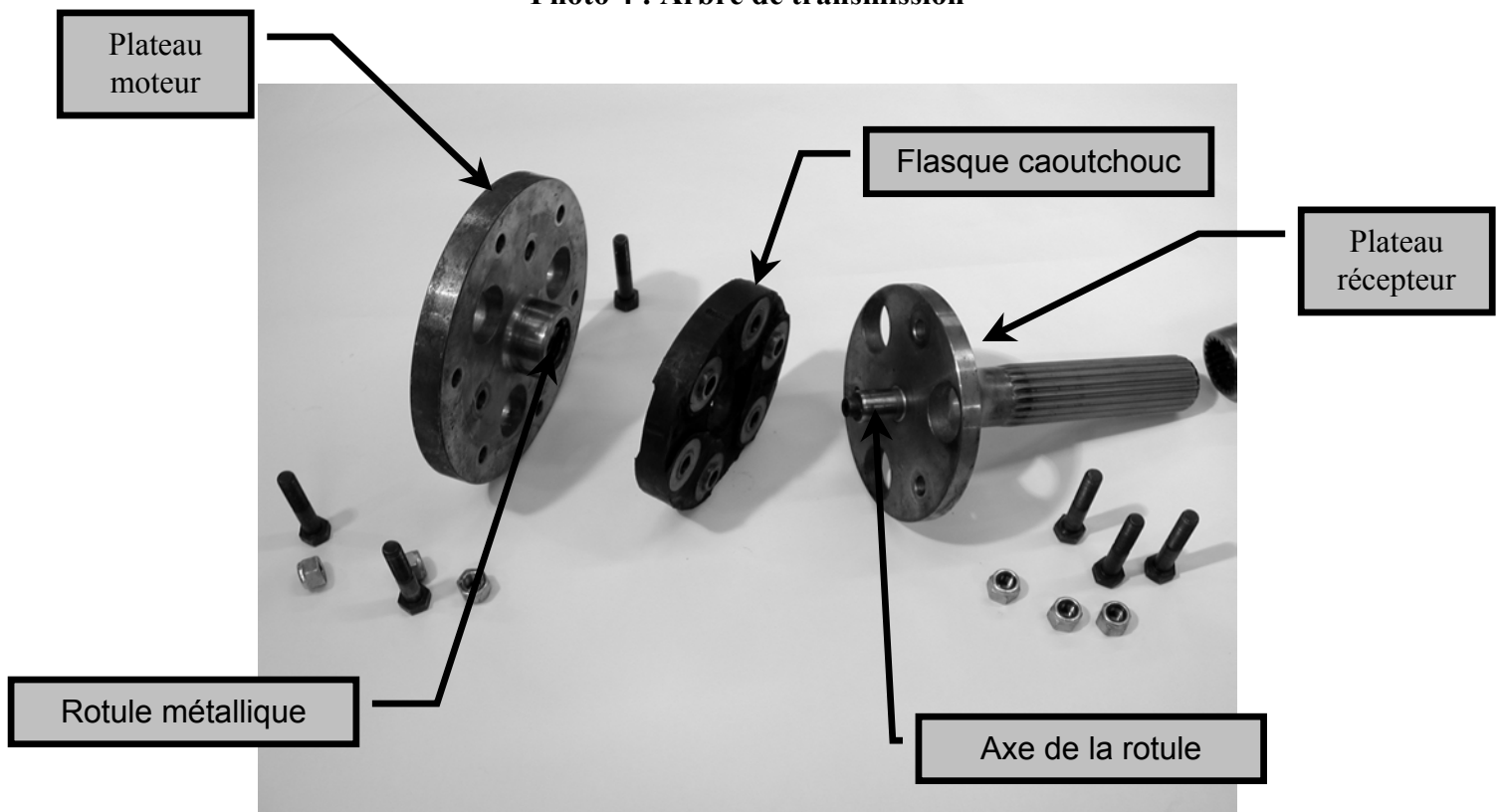
Photo 4 : Arbre de transmission
